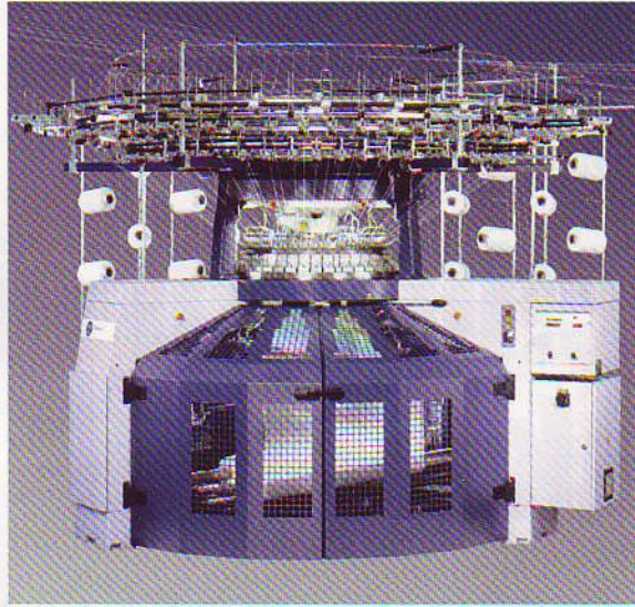
Terrot S296-1 in Breitwickelaus- führung
